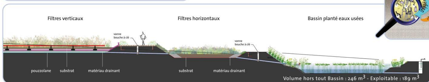
Schéma de traitement des eaux pluviales et usées
